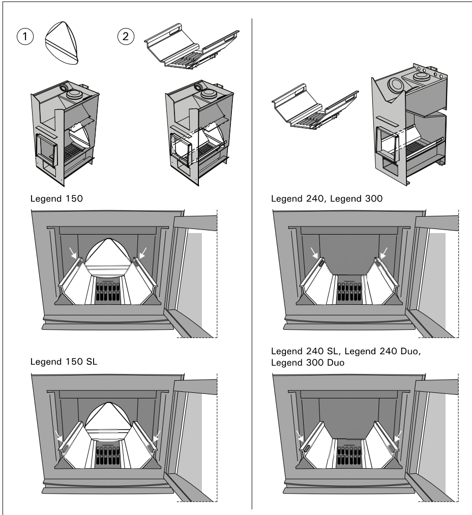
Figure 2. Combustion air channels Abbildung 2. Verbrennungsluftkanäle
