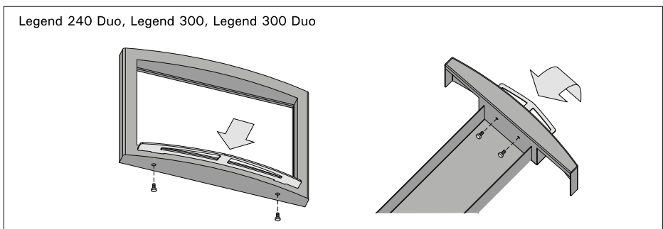
Figure 16. Installing the handles Abbildung 16. Installieren der Griffe
