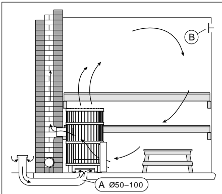
Figure 6. Gravity exhaust ventilation Abbildung 6. Schwerkraftentlüftung
