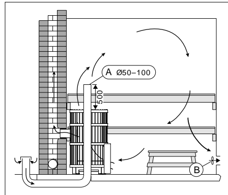
Figure 7. Mechanical exhaust ventilation Abbildung 7. Mechanische Entlüftung
