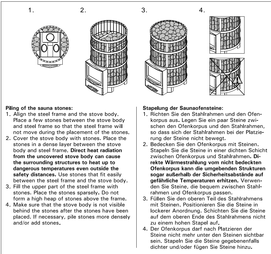
Figure 3. Piling the stones Abbildung 3. Stapeln der Steine
